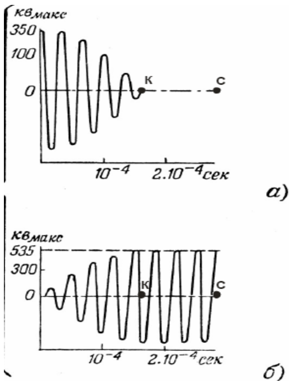
Рис. 4. Осциллограммы колебаний напряжения в катушке Тесла: а) в первичной обмотке, б) во вторичной.
